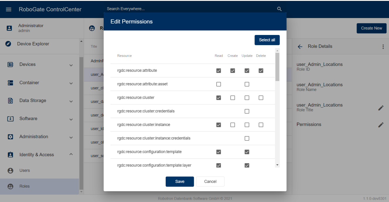
Abbildung 40. Zuweisen oder Entfernen von Zugriffsrechten einer Rolle auf die Ressourcen des ControlCenter
