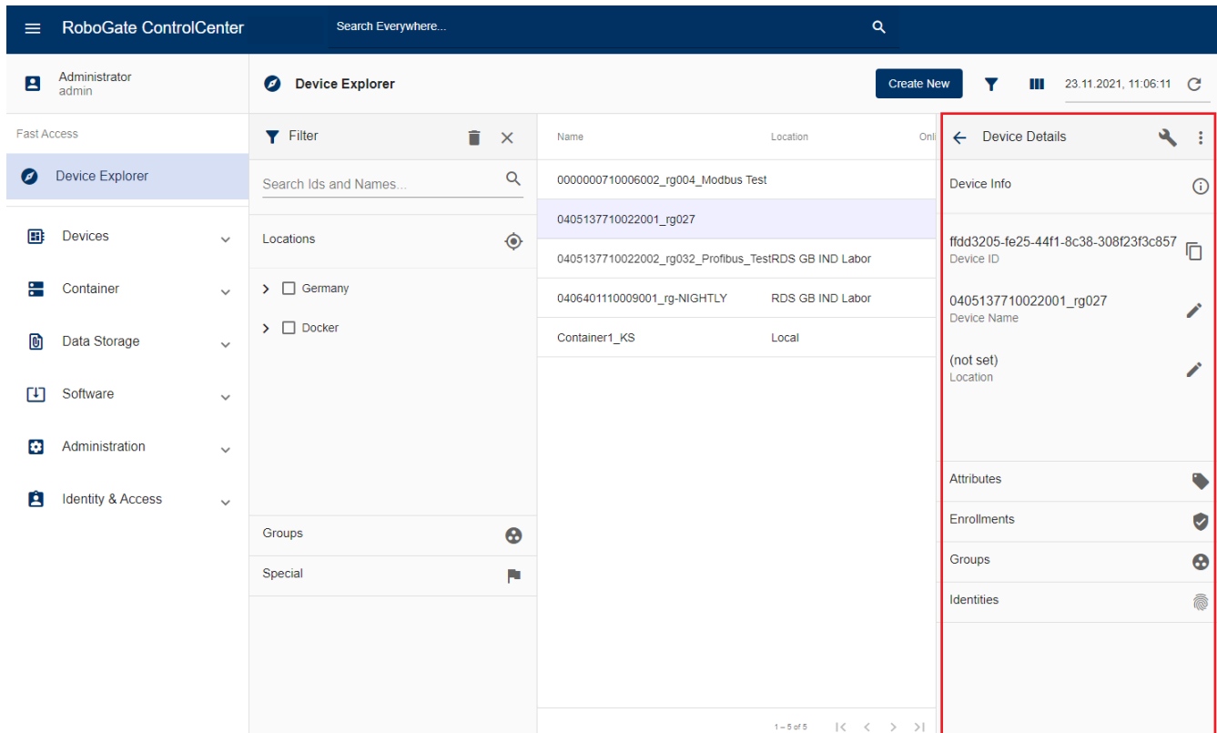
Abbildung 4. Device Explorer mit Ansicht der Detailinformationen des ausgewählten Devices
