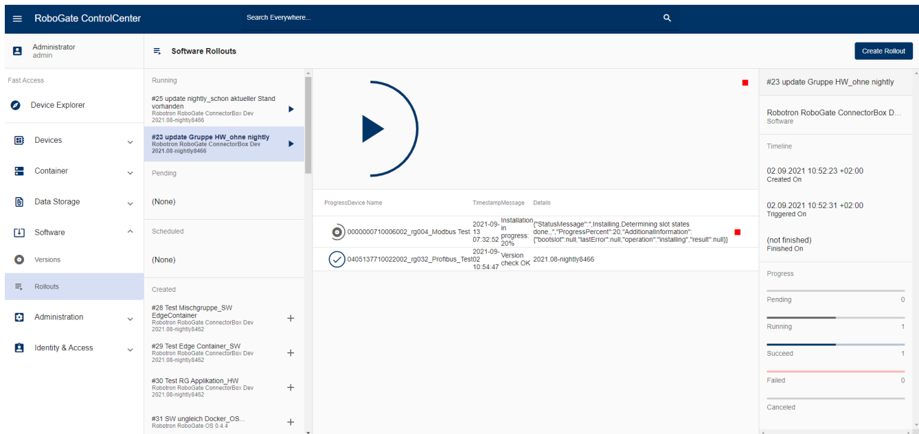
Abbildung 28. Übersicht und Status der Software Rollouts
