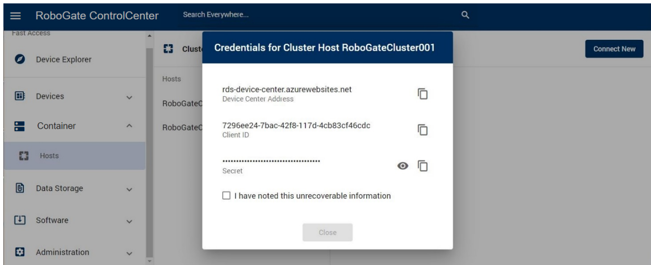
Abbildung 22. Informationen des neu erstellten Cluster Host
