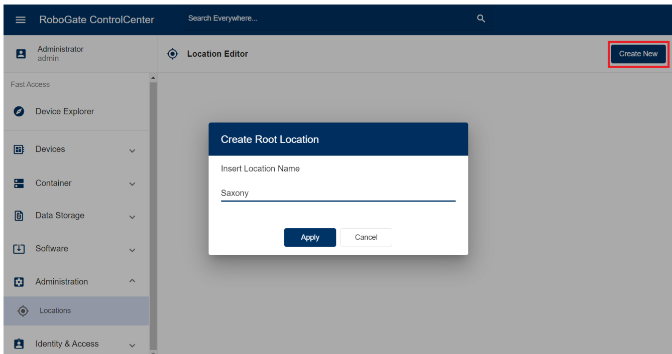
Abbildung 33. Erstellen eines neuen Standorts
