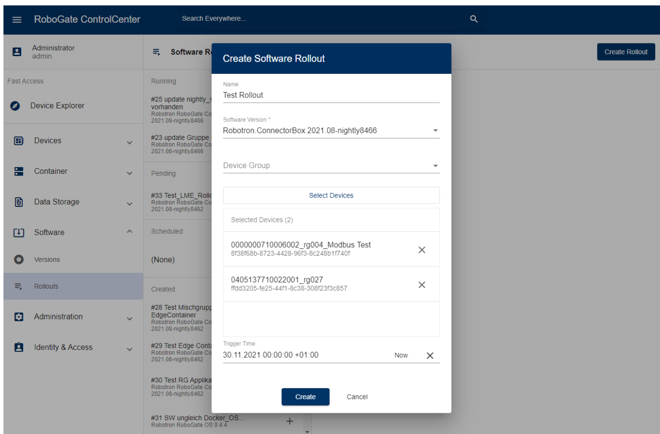
Abbildung 29. Erstellen eines Software Rollout
