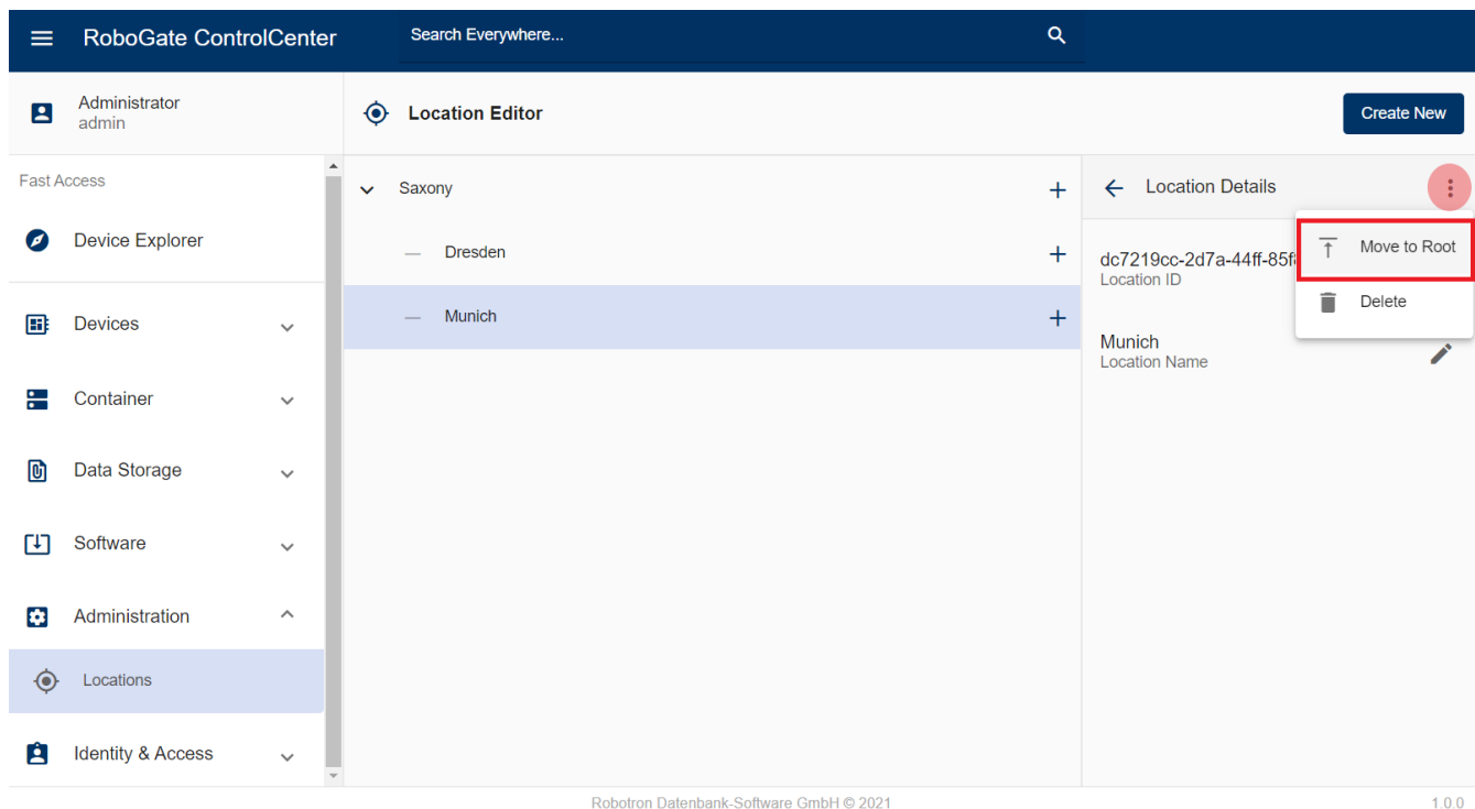
Abbildung 35. Definition eines Unterstandorts als Hauptstandort
