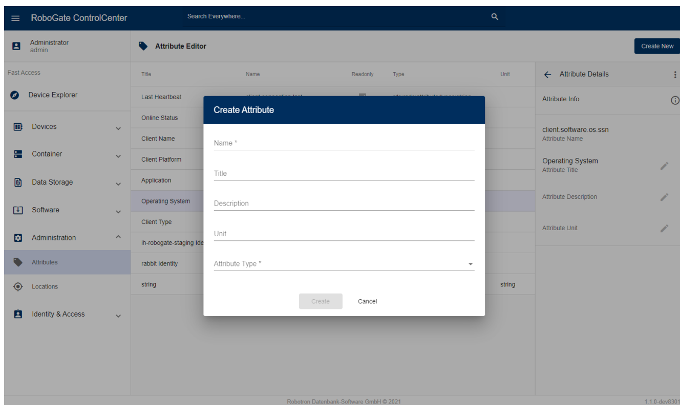
Abbildung 31. Ein neues Attribut erstellen
