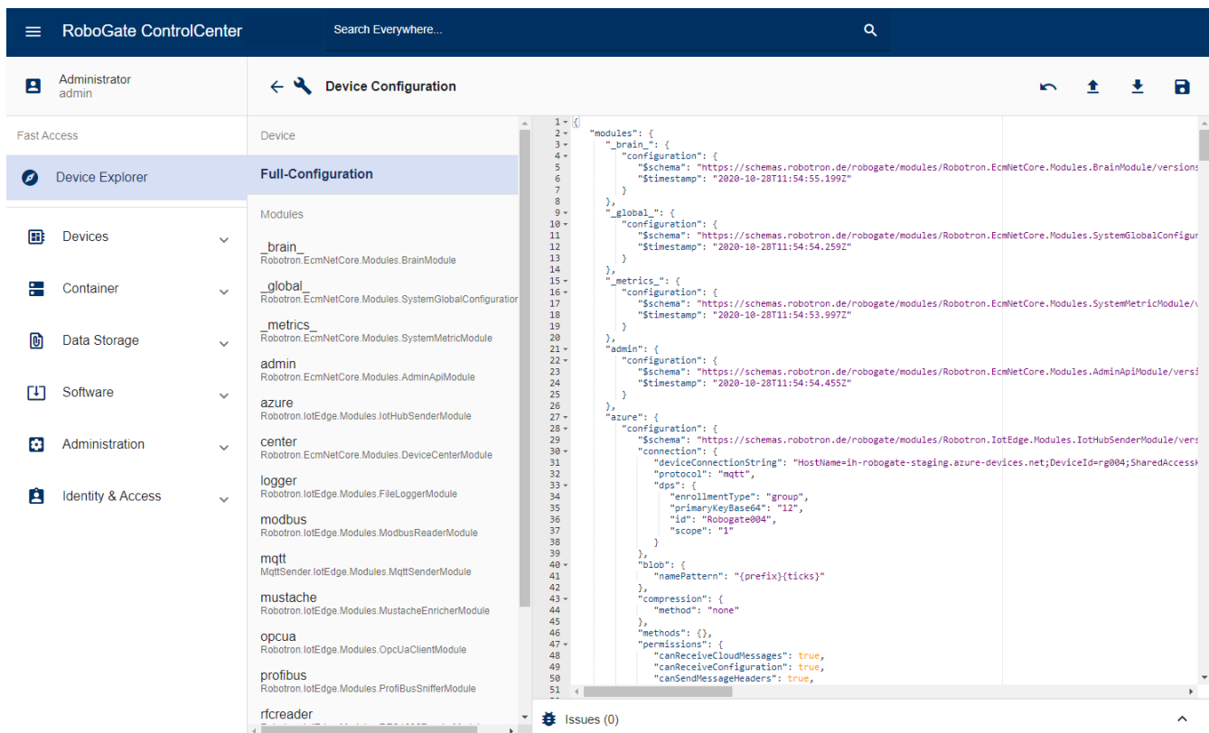
Abbildung 7. Device Configuration des ausgewählten RoboGate Edge
